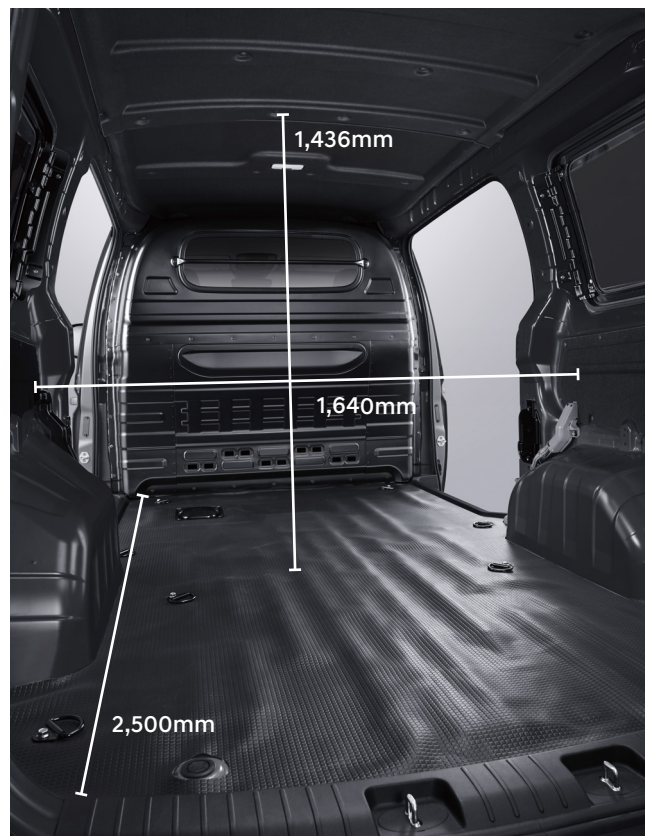
三座佈局的載貨空間 3-seater cargo space
