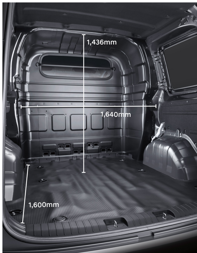
六座佈局的載貨空間 6-seater cargo space
